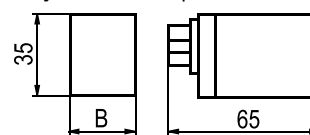
Рисунок 2. Реле с розеткой типа 1
