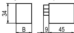
Рисунок 1. Реле без розетки
