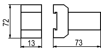
Рисунок 3. Реле с розеткой типа 2
