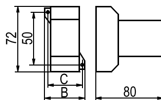
Рисунок 4. Реле с розеткой типа 3
